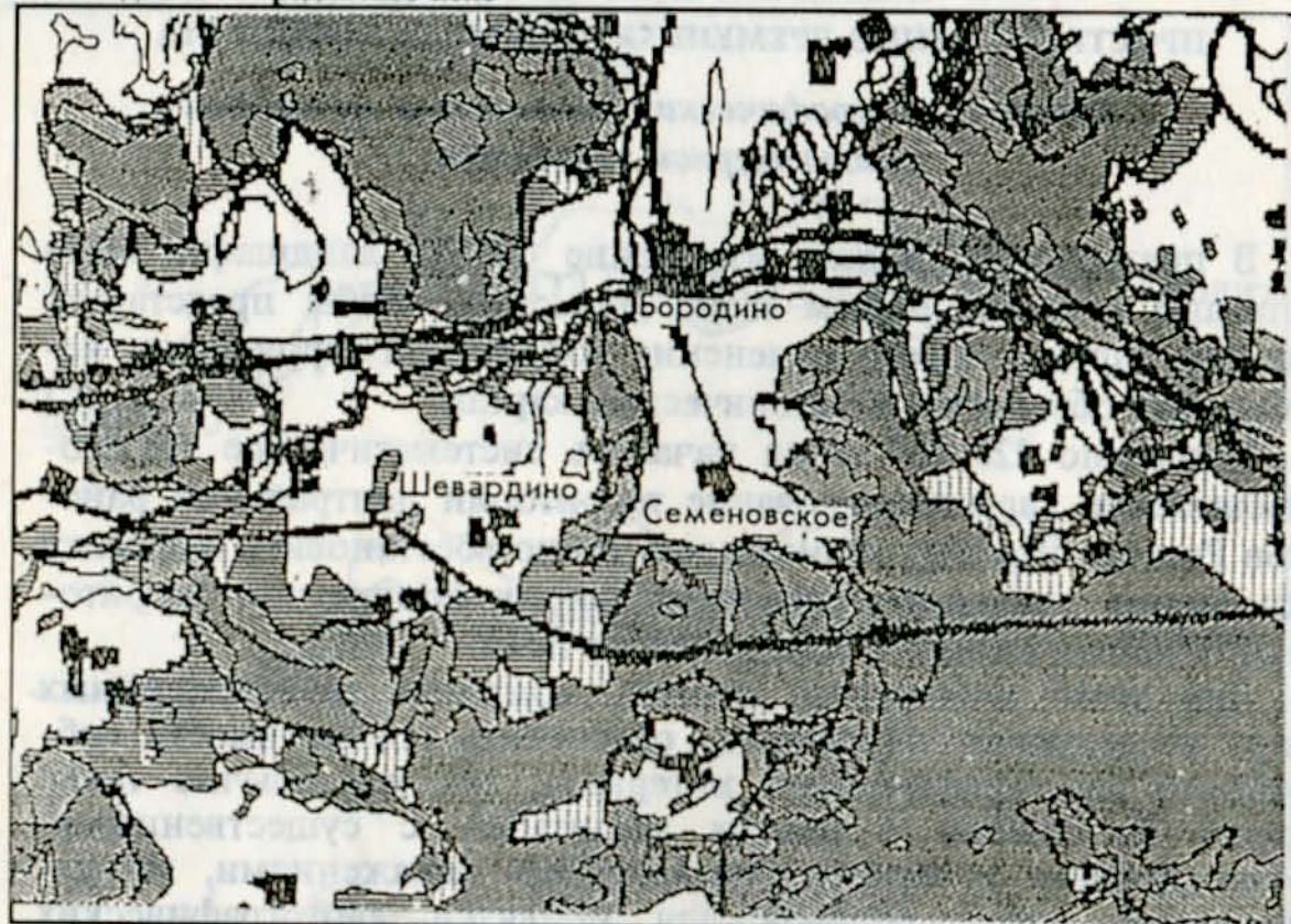
Рис.2. Карты исторической динамики угодий территории Государственного музея-заповедника "Бородинское поле"
