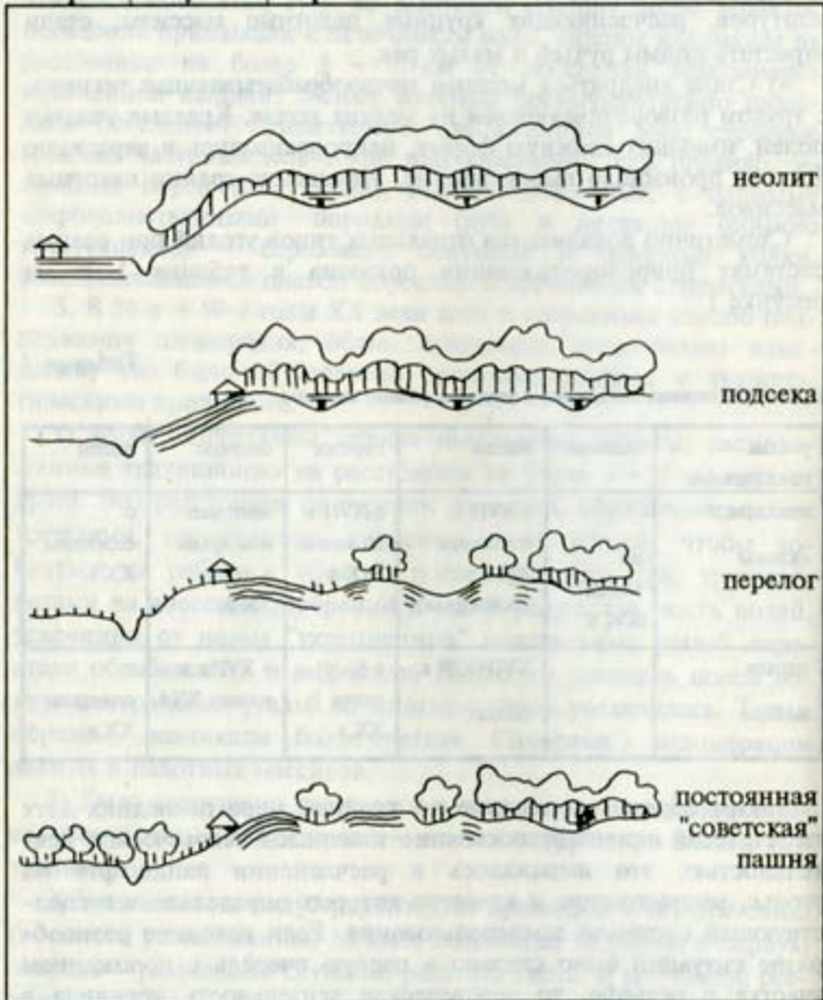
Рис.1 Изменение облика ландшафта за исторический период
